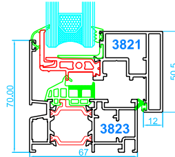
Marco Estándar Hoja de ventana reforzada
