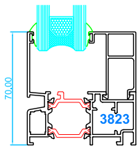
Marco para fijo
