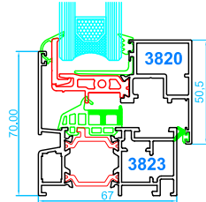
Marco Estándar Hoja de ventana
