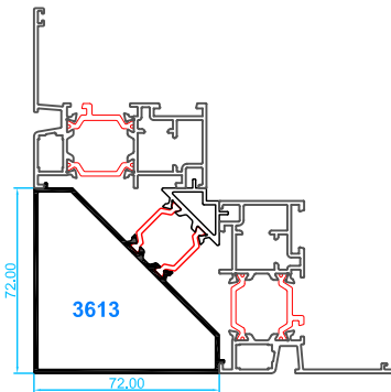
Esquinero de 90°
