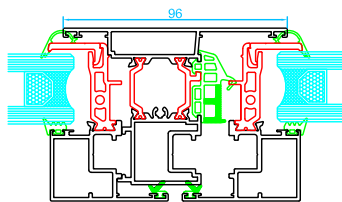
Unión hoja nudo central
