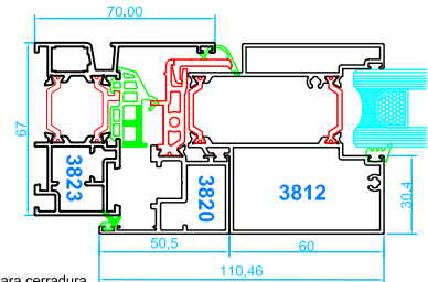
Hoja con acople para cerradura
